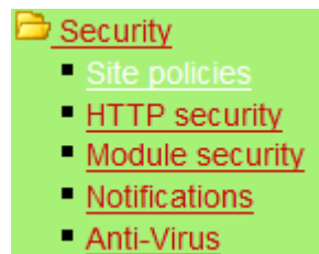
Gambar 20. Pengaturan keamanan
